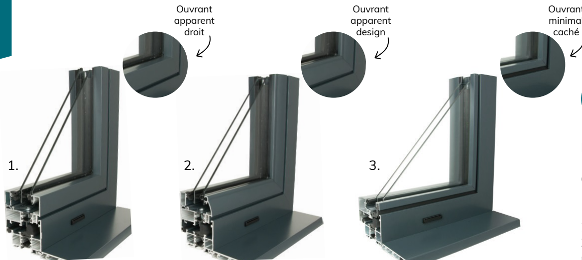
Rupture de pont thermique pour une isolation maximale - Double vitrage à isolation renforcée
