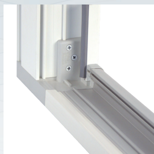
SEUIL ALU À BATTEMENT À RUPTURE THERMIQUE
