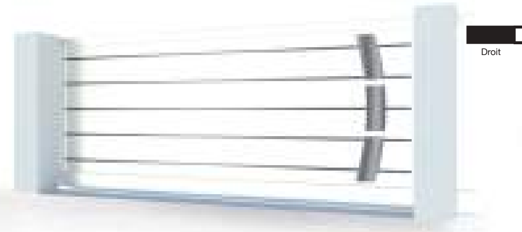
PORTAIL THAR — Coloris : RAL 9016 FT - Lames Horizontales 240 (ou lames 150) - Lames 20 Argentées - Décor N°10 sur les 2 faces -
